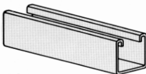
PS 300 1 5/8" x 1 3/8" x 12 ga.
